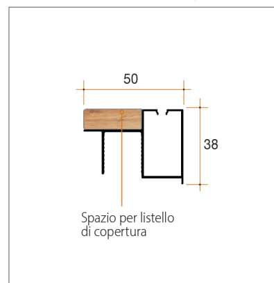
Guida ad incasso soluzione 2 (opzionale)
