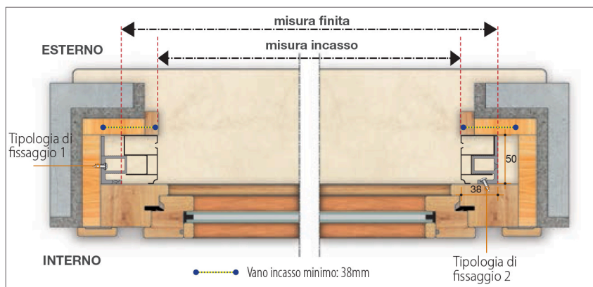
Sezione orizzontale
